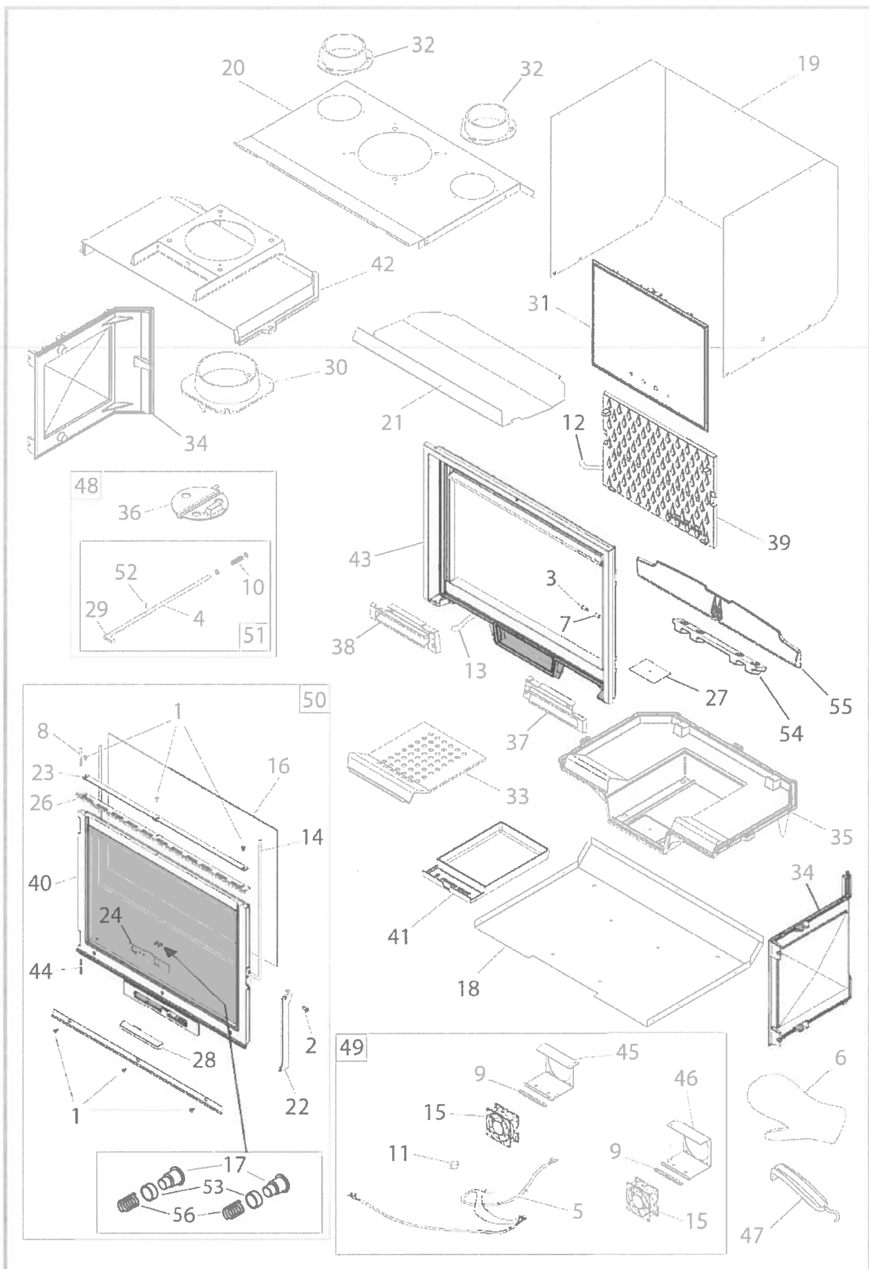
Figuur 19 - Wisselstukken
