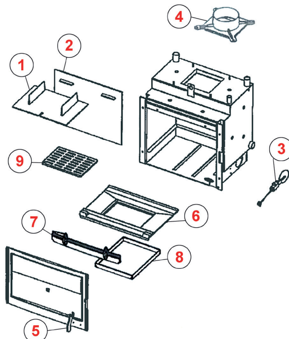
8 CENDRIER ASBAK 1 3316 5152 GO 5152-08
